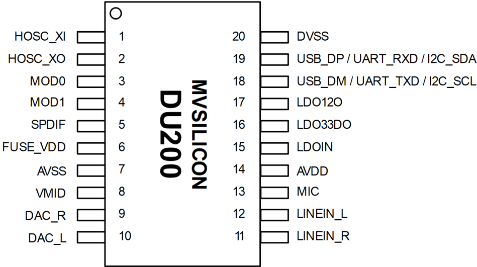
图 2. 芯片引脚定义
