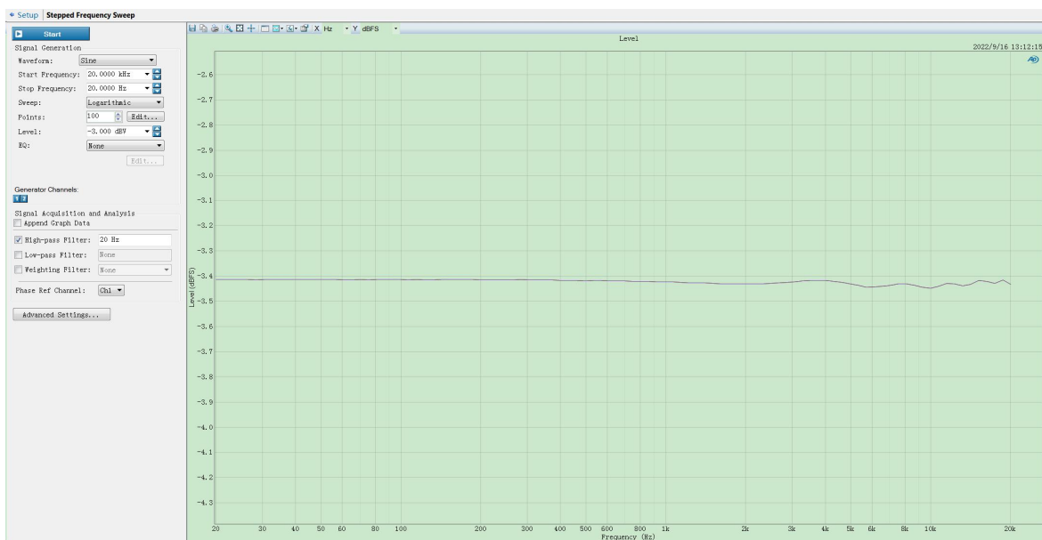
图 3，频响曲线
