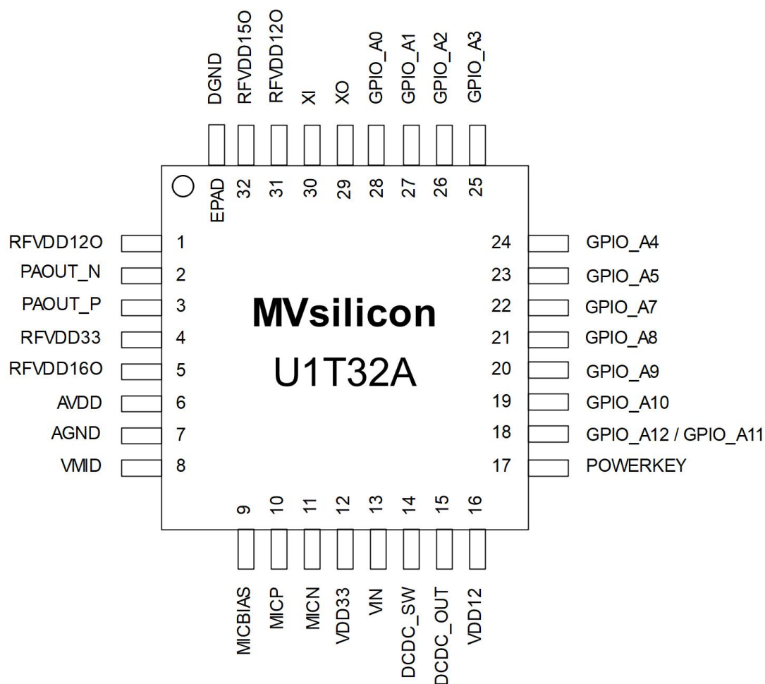
图 1，封装引脚示意图（QFN32-5x5mm）
